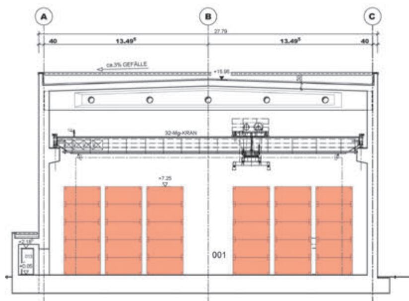
Schnitt eines von der WTI geplanten Lagergebäudes.
