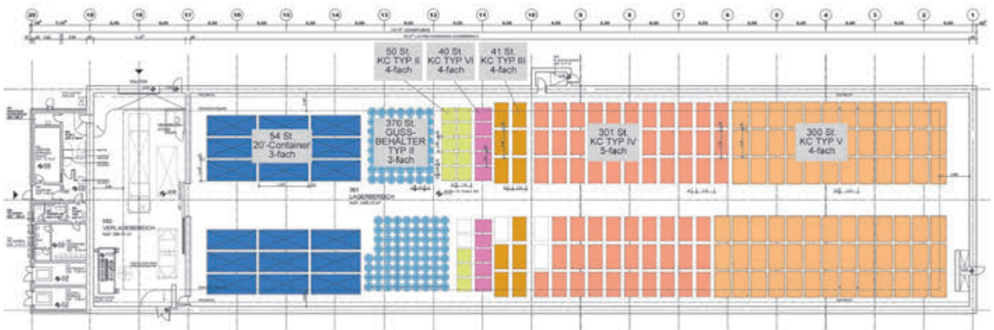
Grundriss eines von der WTI geplanten Lagergebäudes.
