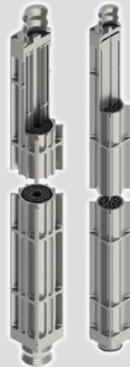
Die Köcher für Brennstäbe aus DWR- (links) und SWR-Anlagen.
